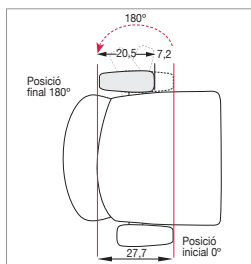
Moviment Pivotant 180 ° del braç que permet el gir en sentit horitzontal del reposa-braços
