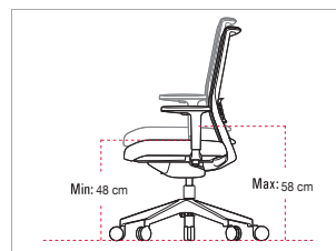
Altures màximes i mínimes del seient
